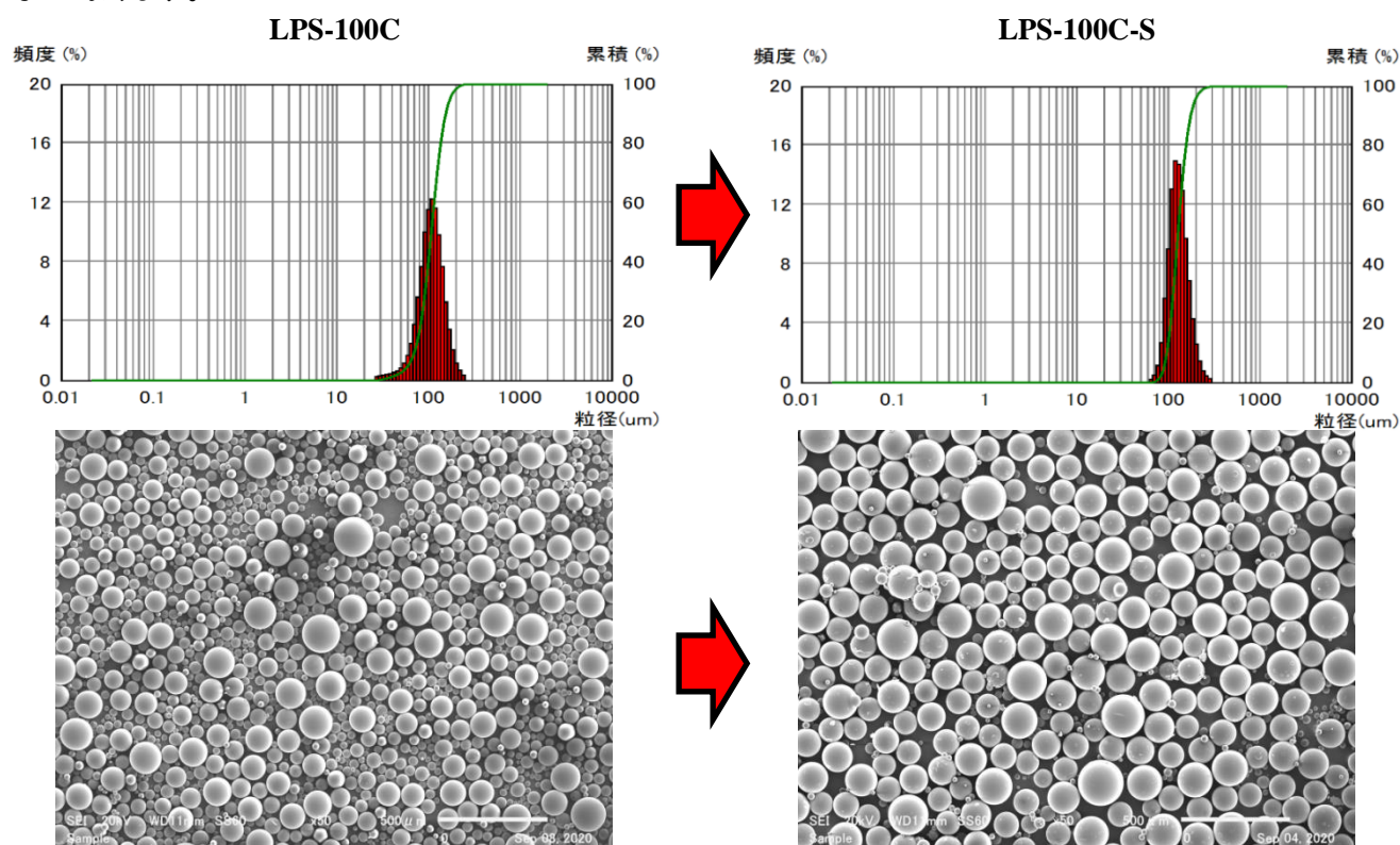
【LPS-S の製品一例】
